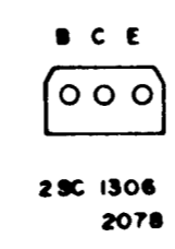
2SC 1306 2078
