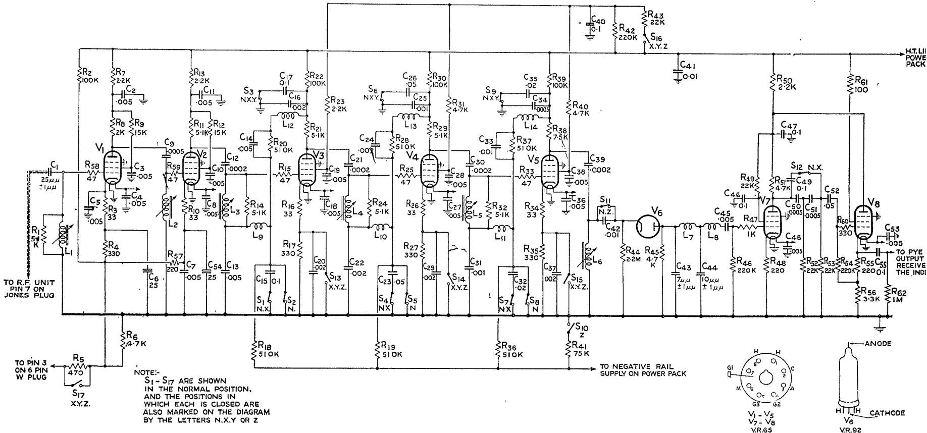
Fig. 20.—R.1355, IF amplifier circuit.
