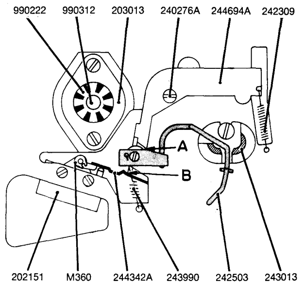
Fig. 4.35 Neutral.
