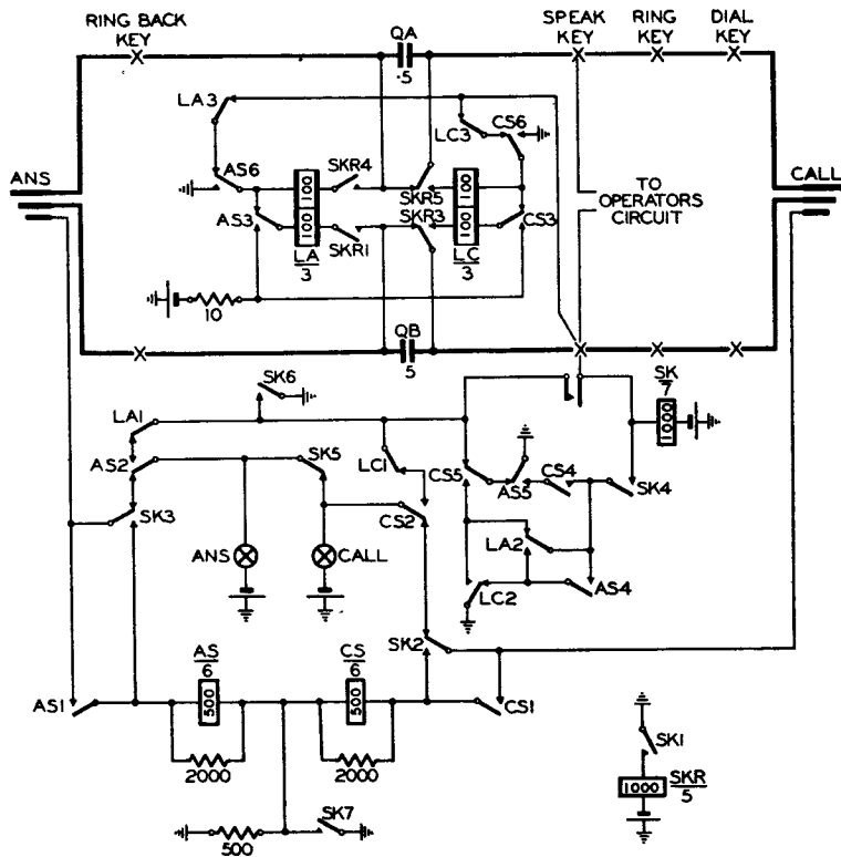
FIG. 6.—CORD CIRCUIT.
