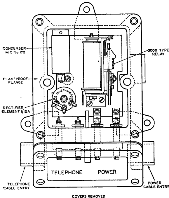
FIG. 6.—RELAY UNIT.
