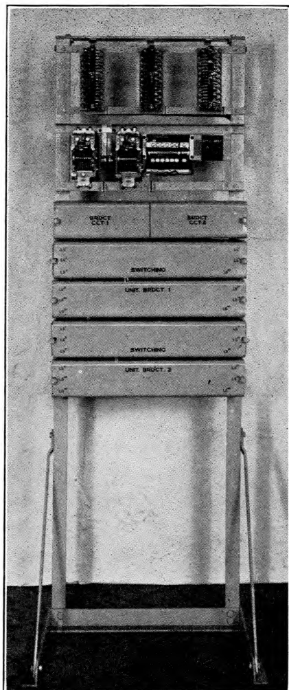
FIG. 2.—SWITCHING UNIT.
