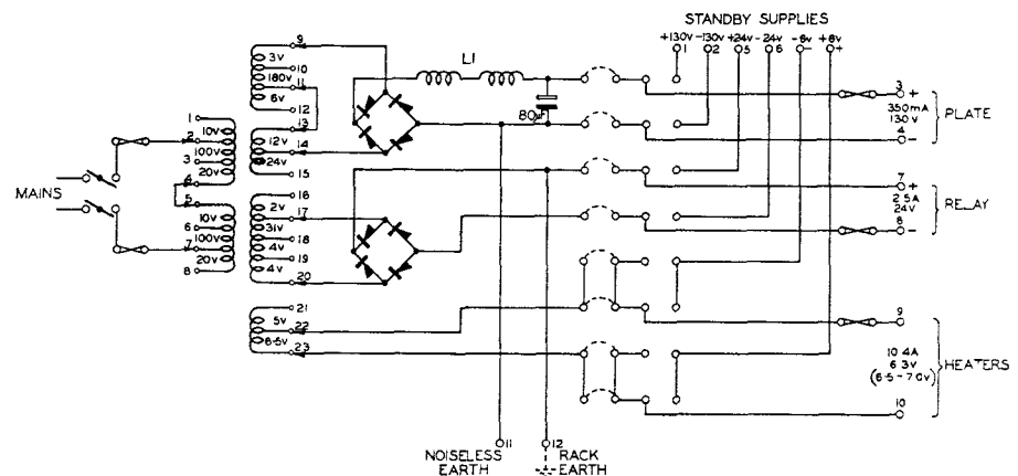
FIG. 5.—MAINS UNIT.
