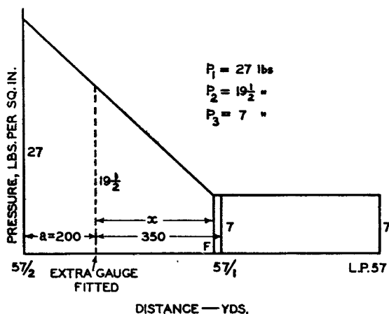
FIG. 2.—TYPE "B" FAULT.
