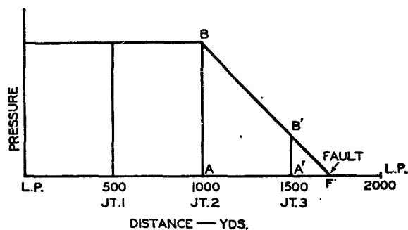
FIG. 1.—TYPE "A" FAULT.
