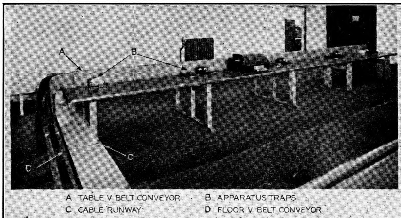
FIG. 5.—INSTRUMENT TABLES.
