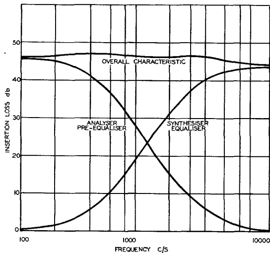
FIG. 4.—SPECTRUM EQUALISATION.
