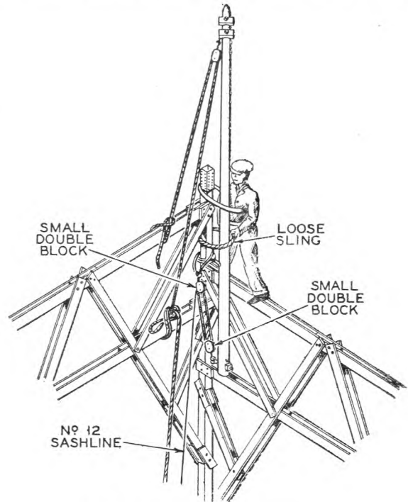
FIG. 5.—LOWERING A DERRICK.
