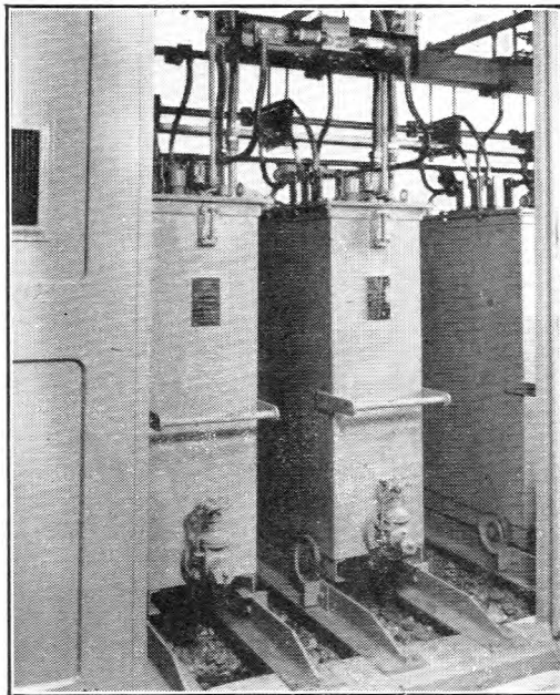
FIG. 6.—RECTIFIER TANK UNITS.
