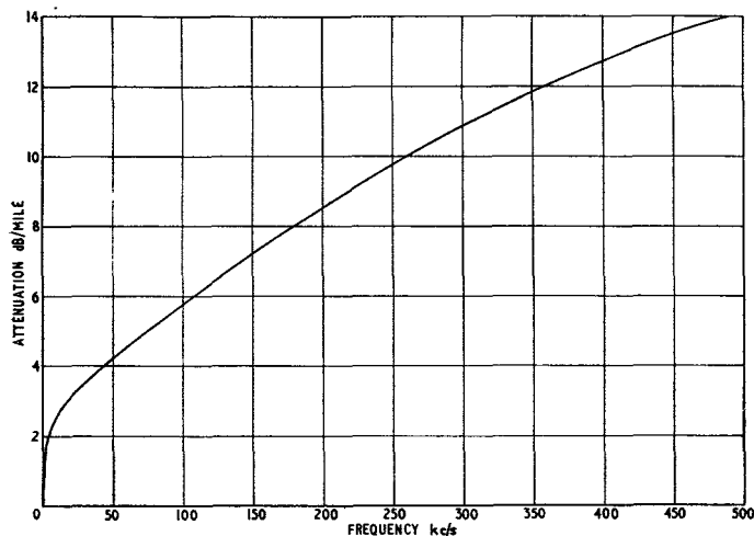
FIG. 2.—ATTENUATION OF 20-LB P.C.Q.T. CABLE
