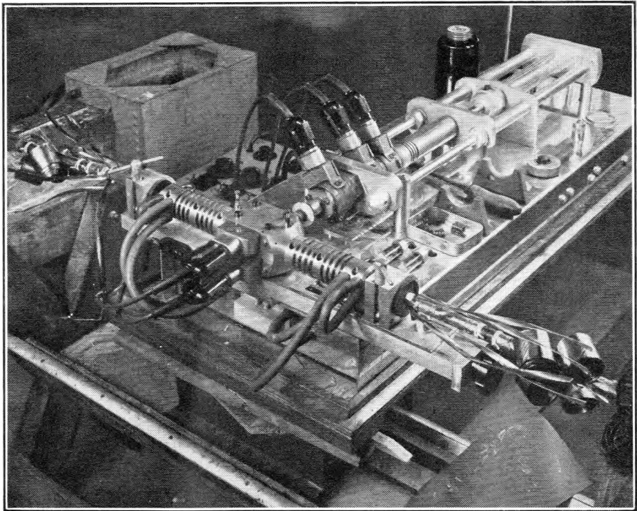
FIG. 3.—POLYTHENE-MOULDING MACHINE.
