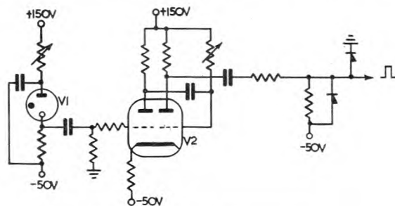
FIG. 9.—120-P.P.S. GENERATOR.
