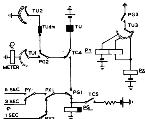
FIG. 3.—TIMING CIRCUIT.
