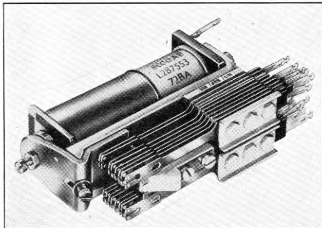
(d) Post Office 3000-Type Relay.
