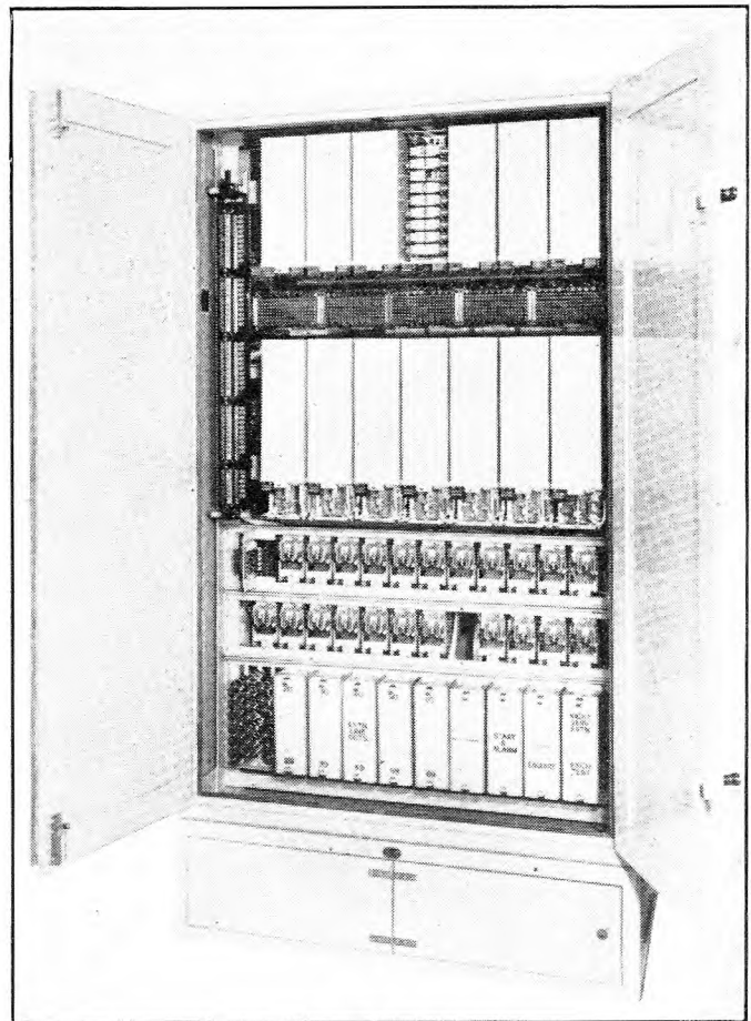
FIG. 19.—P.A.B.X. No. 1.
