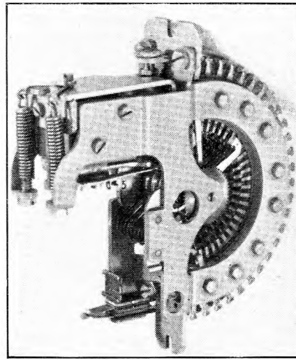
(d) Post Office Unisector No. 3.
