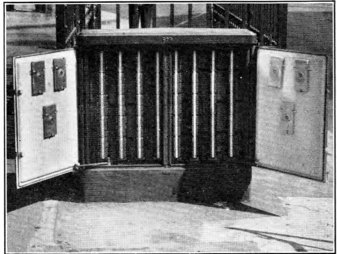
FIG. 13.—CROSS-CONNEXION CABINET.
