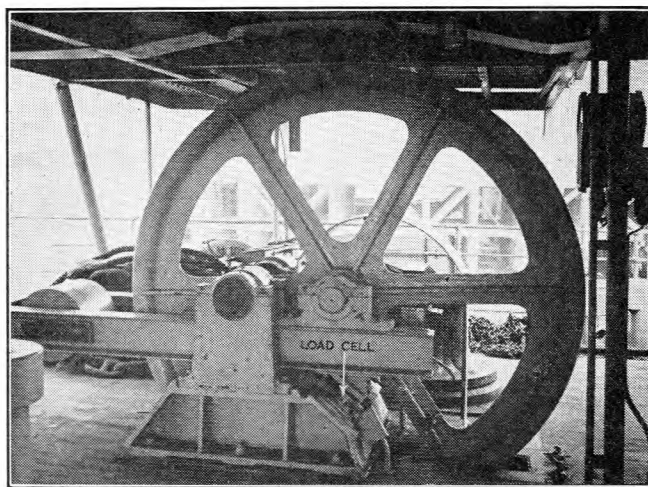
FIG. 3.—DYNAMOMETER SHEAVE.
