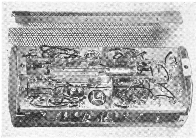
FIG. 5.—AMPLIFIER.
