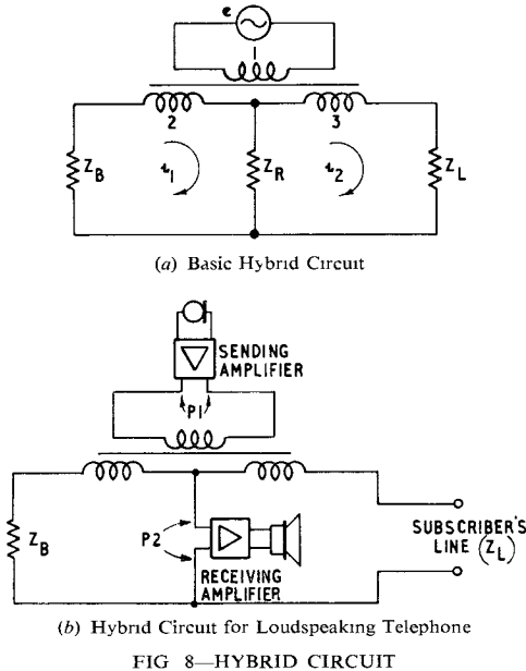
FIG. 8—HYBRID CIRCUIT
