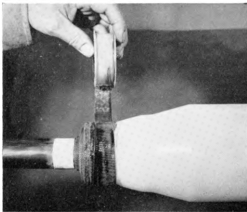
FIG. 6—RESINWRAP JOINT
