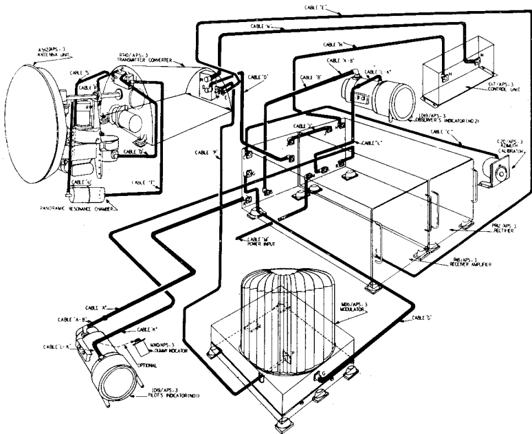
A.S.V. Mark VIII A (A.S.D.1)
