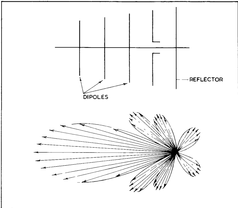
Yagi Array
